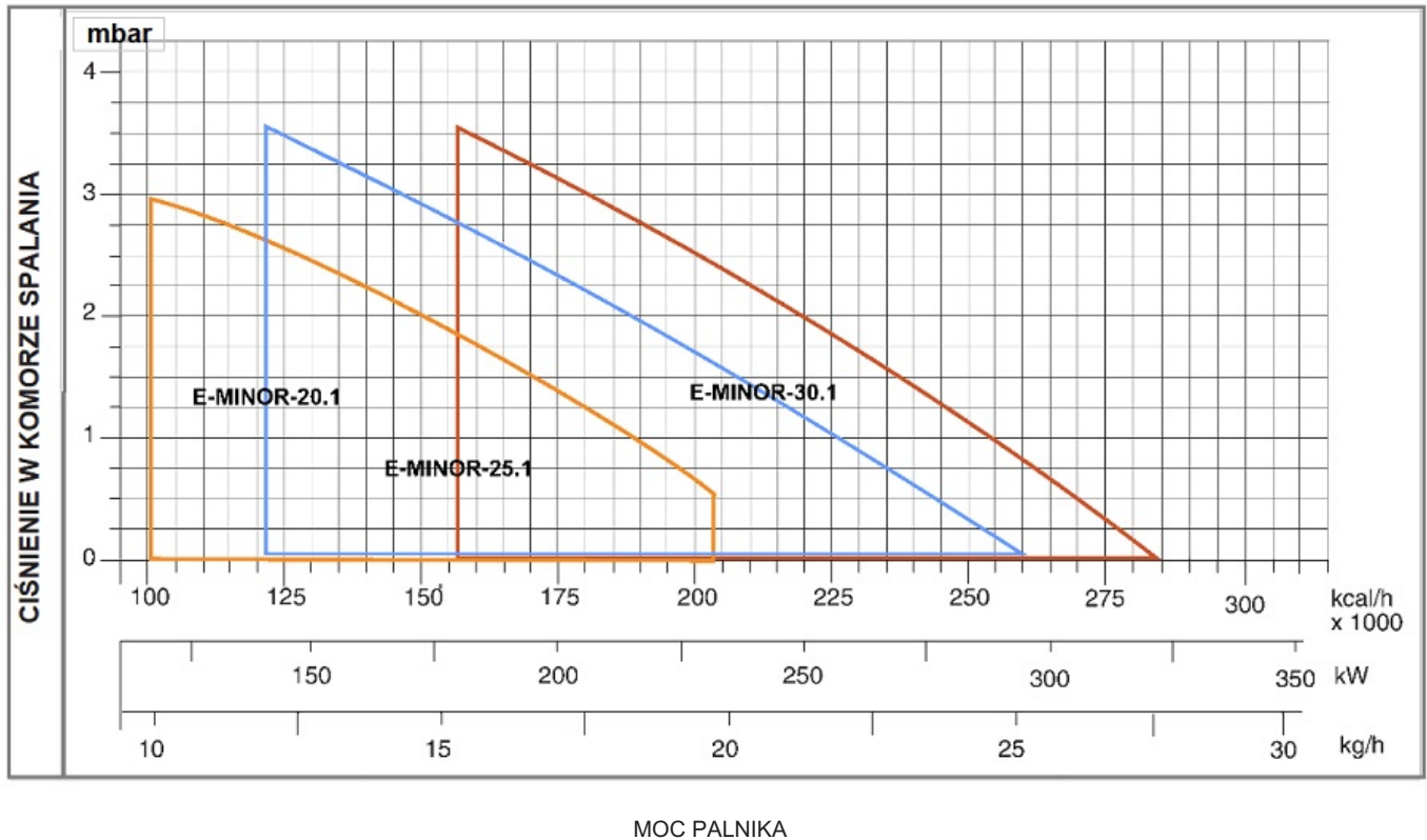
Wykres mocy palnika ( 100-204kW, 121-260kW, 156-279kW ) oraz zużycia oleju opałowego (w kg/h) w zależności od ciśnienia w komorze spalania w palnikach Eacoon seria MINOR 20.1/25.1/30.1 .
