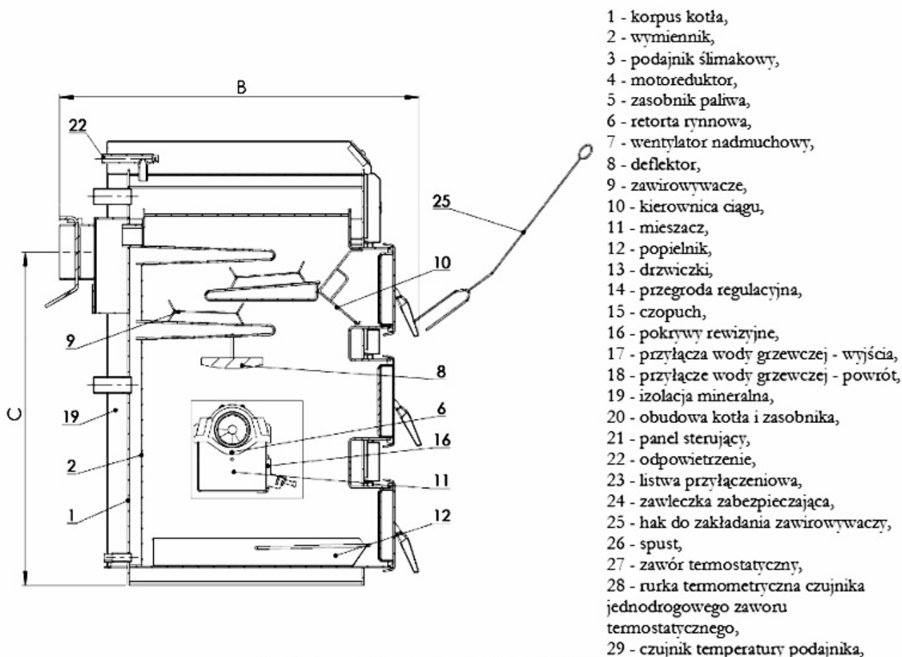
Rys.1 Schemat konstrukcji kotła EKO-KWP multi
